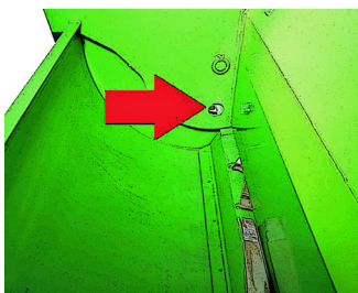
Schmierung im Pressraum Lubrication inside the compaction chamber
