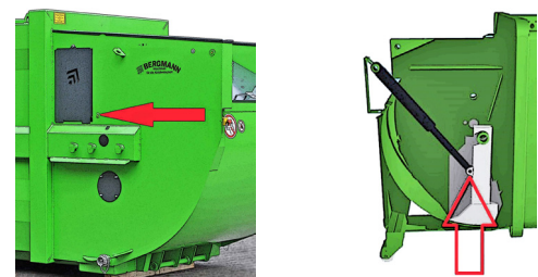
Schmierung außen erreichbar. Kein Einstieg in den Pressraum erforderlich. Lubrication accessible from outside. No need to enter the compaction chamber
