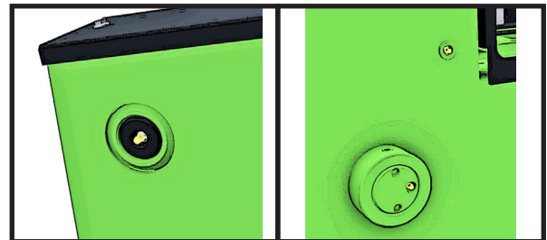
sämtliche Schmierstellen sind von außen zugänglich, auch innenliegenden Kolben all greasing points can be reached from the outside, also the inside piston
